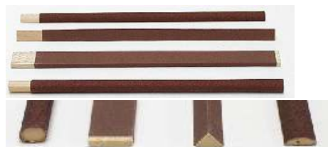
Schuurstokken : lengte 210 mm. Cabrons en papier d' émeri : longueur 210 mm.
